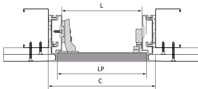
CARTONGESSO - DOPPIA LASTRA
