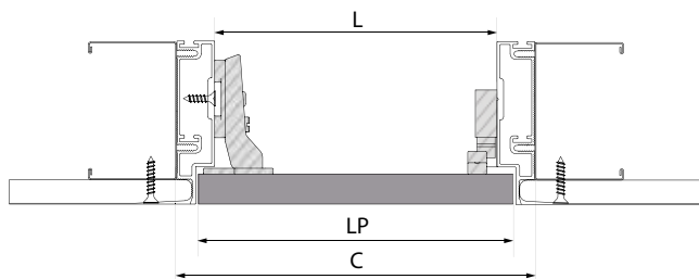
CARTONGESSO - UNA LASTRA
