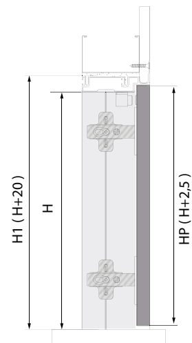
CARTONGESSO - 3 LATI
