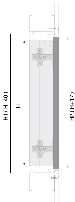
CARTONGESSO - 4 LATI
