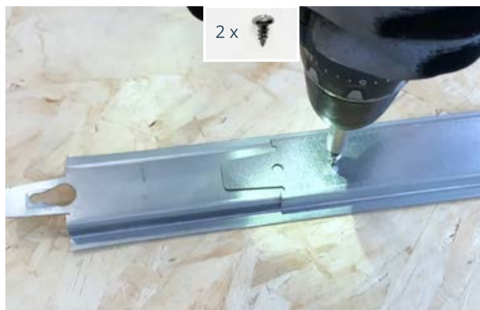
Fissa le estremità dei distanziali con delle viti. Fix both spacers end by screws.
