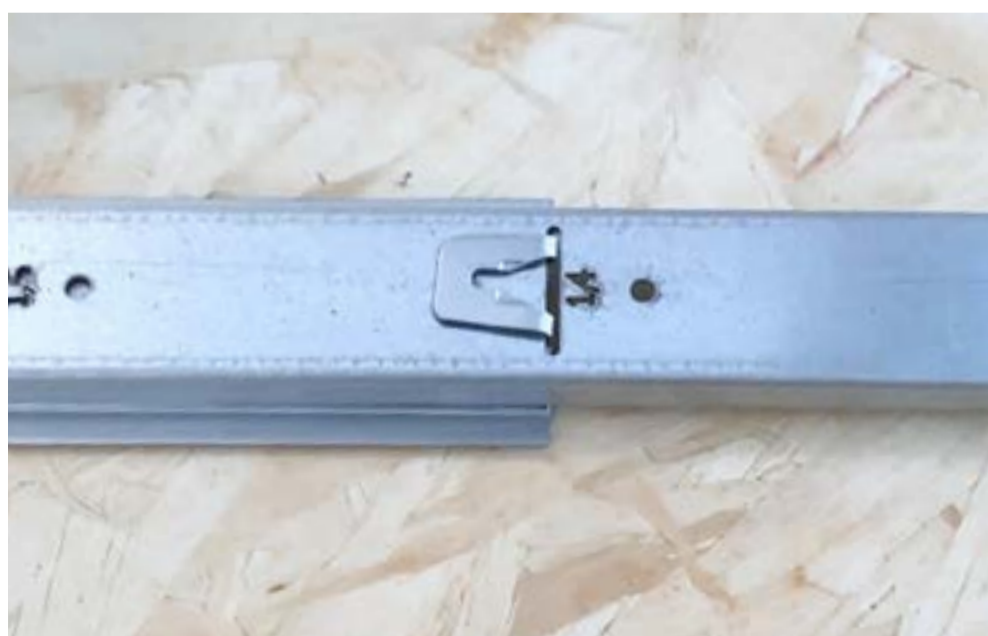
Ripiegare la linguetta dei distanziali per fissarli. Fold on itself the spacer tab in order to fix them. Do it for both spacers.
